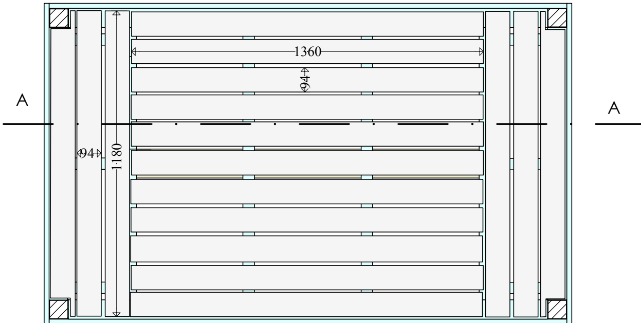
Schnitt B - B mit Bretter
