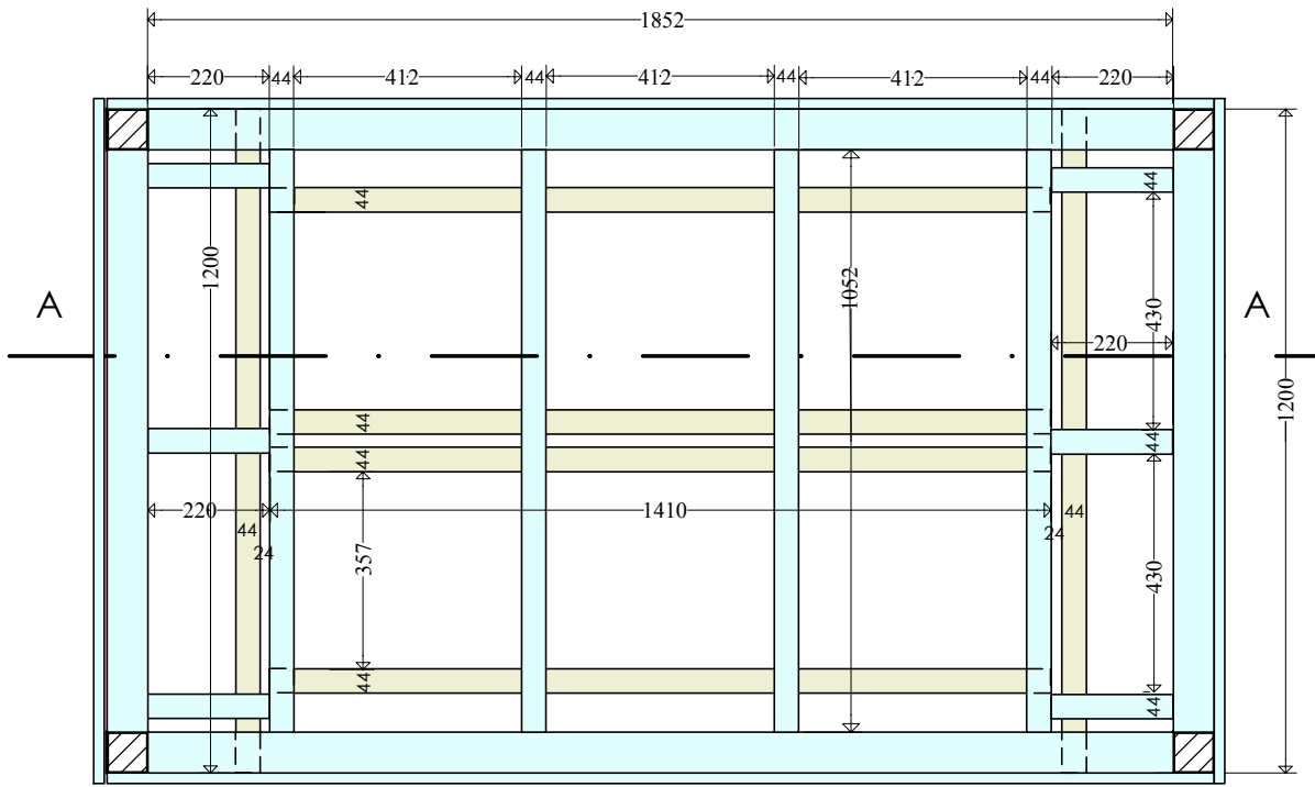
Schnitt B - B ohne Bretter
