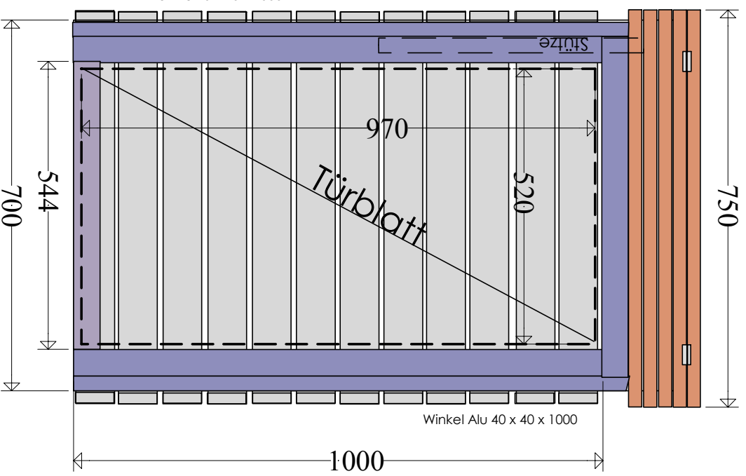
Frontansicht (Abdeckwinkel nicht dargestellt)
